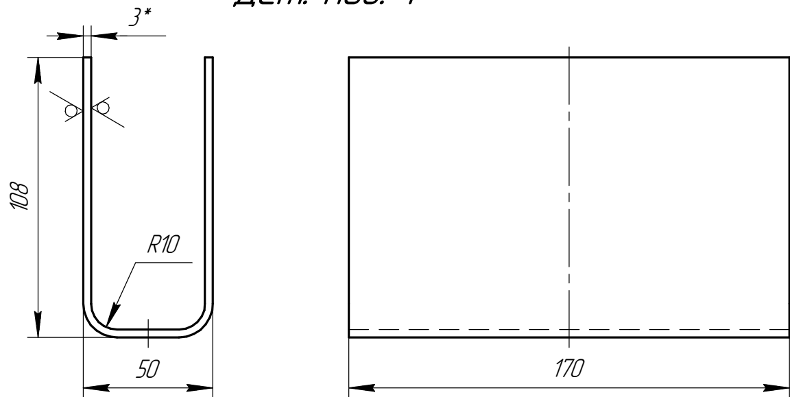
Дет. поз. 1
